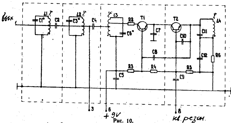
Рис. 10. Схема электрическая принципиальная гетеродина
